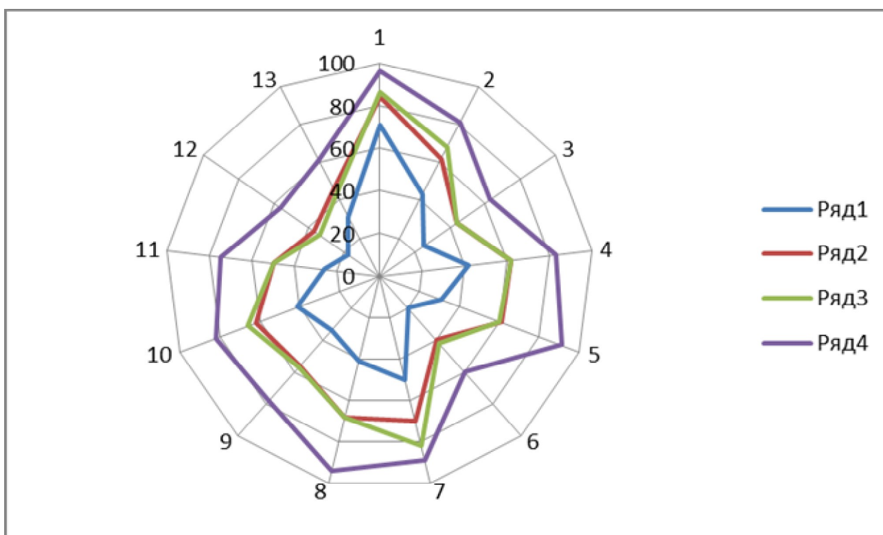
Рис. 2. Положение синтаксонов кекуров на градиентах факторов среды.
